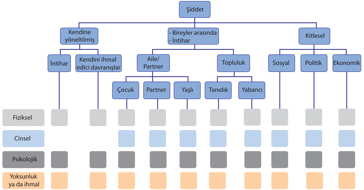
Şekil 6.1 Şiddet Tipolojisi
