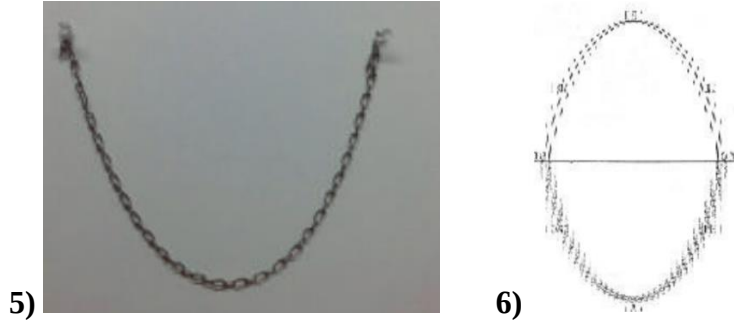
Şekil 5: İki nokta arasında asılı duran ve yalnızca kendi ağırlığıyla yüklenen zincirlerle oluşturulan zincir veya fönüküler eğri (Chilton ve Tang, 2016).
