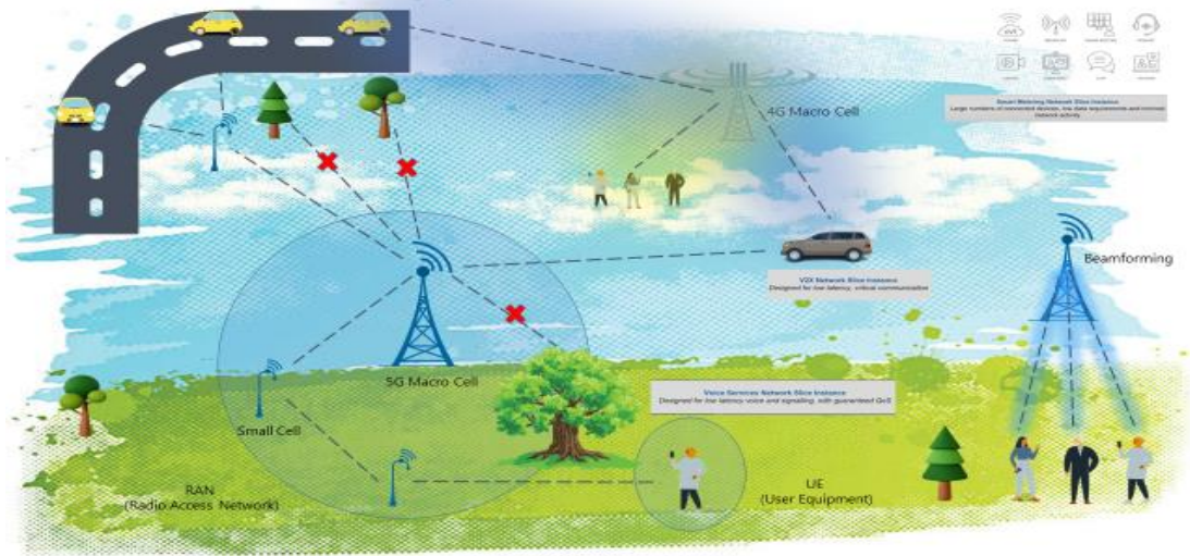
Şekil 1.2: 4G ve 5G Bağımsız Olmayan Dağıtım (NSA)
