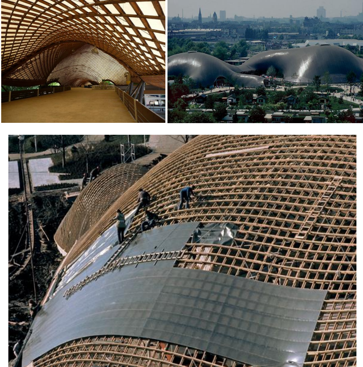
Şekil 10: Bundesgartenschau ızgara kabuğunun iç ve dış mekân görünümleri, (Hafif Yapılar ve Kavramsal Tasarım Enstitüsü [ILEK], 1975).
