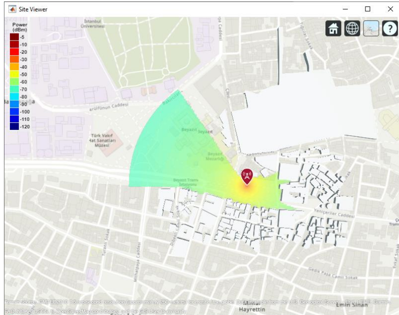
Şekil 2.1: Maksimum Yansıma Sayısını 0 Kabul Eden Kapsama Haritası Kaynak: Matlab
