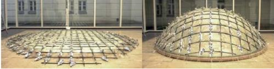
Şekil 12: Şişirme ile yükseltme yöntemi (Quinn, Gengnagel ve Williams, 2015).
