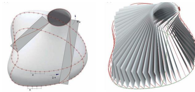
Şekil 7: Hermes, Rive Gauche, Paris – serbest biçimli ahşap ızgara kabuğu pavyonlarının parametrik tasarım yazılımları kullanılarak çizilmiş formları; üç kontur eğrisinin düzgün segmentlere bölünmesi ve seçilen ofset düğümlerinin bağlanmasıyla oluşturulan bölümler (Chilton ve Tang, 2016).
