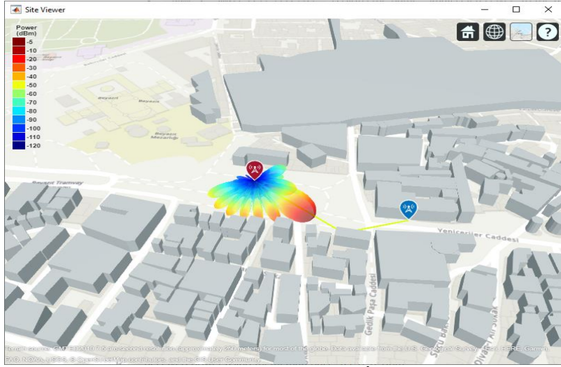
Şekil 3.2: Beam Steering ile İletim Yolu Kaynak: Matlab
