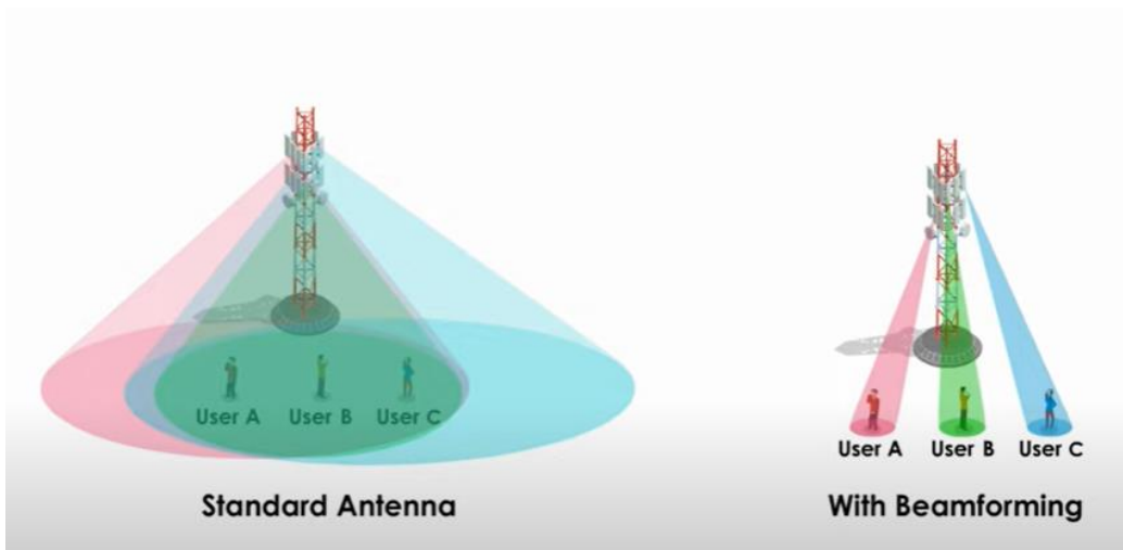
Şekil 1.10: Beamforming ile 5G Hücresel Ağlar Kaynak: Sunny Classroom.
