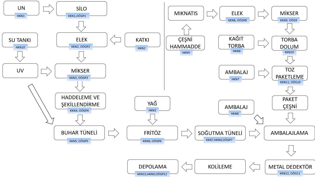
Şekil 1. Noodle Üretim Proses Şeması (Guner & Basdogan, 2024).
