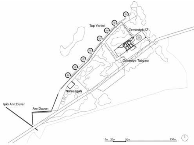
Resim 2:Yer İzi (Atölye Kolektif).
