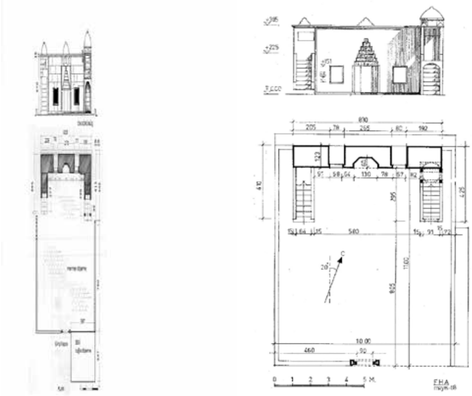
Resim 4: Solda Akmaydalı'nın 22 ve sağda Ayverdi'nin 23 eserlerinde yer alan Gelibolu Azaplar Namazgâhı rölöve çalışmaları.
