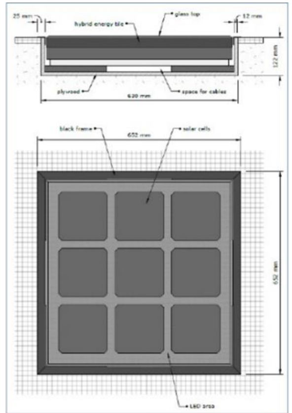
Şekil 5: Piezoelektrik Döşeme
