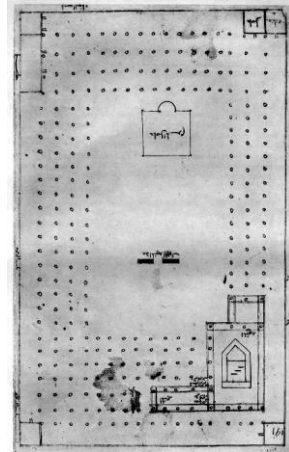
Resim 19. J. Sauvaget'ye göre XV. yy'da [Memluk ilaveli] Mescid-i Nebî'nin tahmini görünüşü
