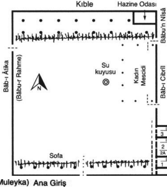
Resim 9b. Mescid-i Nebî'nin Nisan 623'de ilk yapıldığında kiblesi Kudüs (Kuzey) istikametine doğru ve 60x70 zirâ ölçülerindeki hâlinin tahmini krokisi 43
